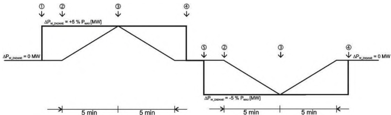
Rys. 2 sprawdzenie działania regulacji wtórnej w odpowiedzi na wymuszenie w torze regulacji wtórnej w trakcie wyłączania i załączania stanu regulacji wtórnej
