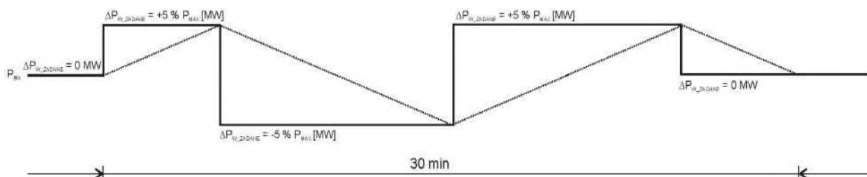
Rys. 4 Sprawdzenie działania regulacji wtórnej w odpowiedzi na wymuszenie w torze regulacji wtórnej w trakcie wyłączania i załączania stanu regulacji wtórnej
