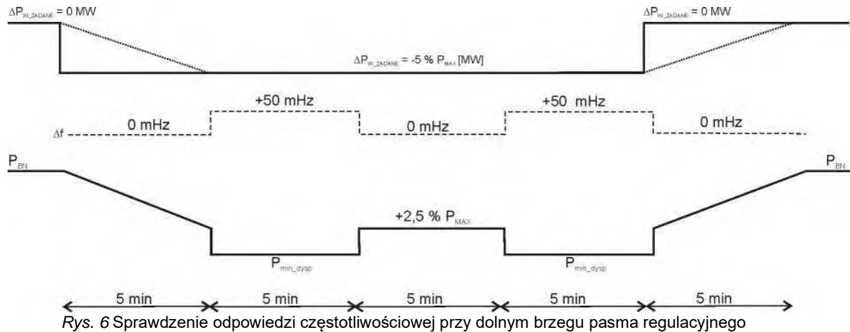
Rys. 6 Sprawdzenie odpowiedzi częstotliwościowej przy dolnym brzegu pasma regulacyjnego
