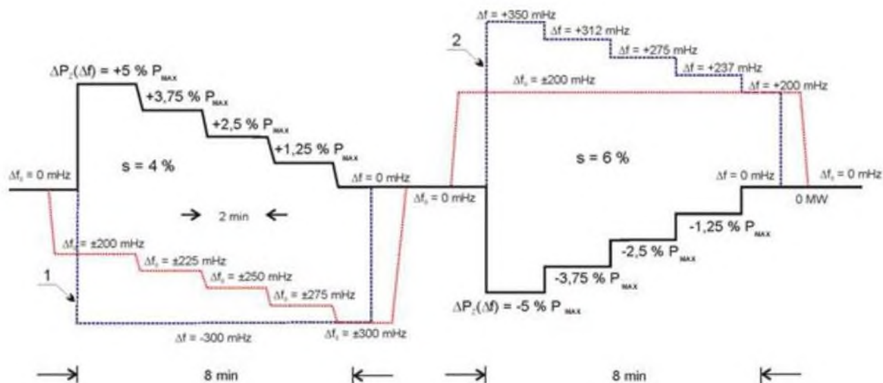
Rys. 4 Sprawdzenie odpowiedzi częstotliwościowej przy zmianach: częstotliwościowej, statyzmu oraz odchyłki częstotliwościowej strefy nieczułości odpowiedzi
