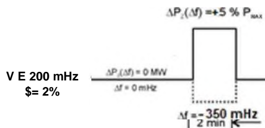
Rys. 2 Sprawdzenie odpowiedzi częstotliwościowej modułu wytwarzania energii w reakcji na symulowaną pełną zadaną odpowiedź częstotliwościową przy przykładowych ustawieniach statyzmu.
